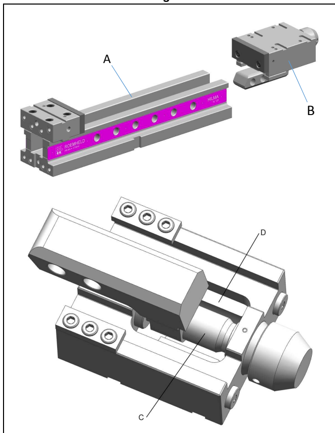
Fig. 8 : Démonter le chariot de serrage
