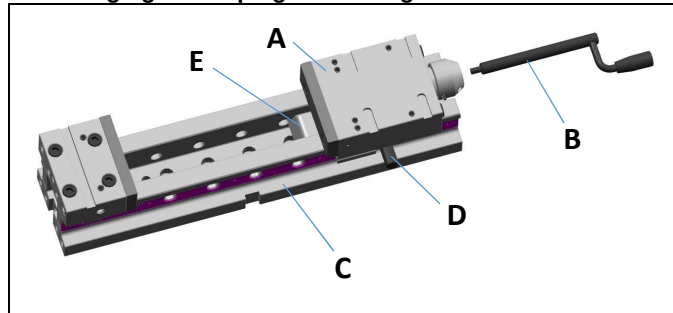
Fig. 4 : Réglage de la plage de serrage
