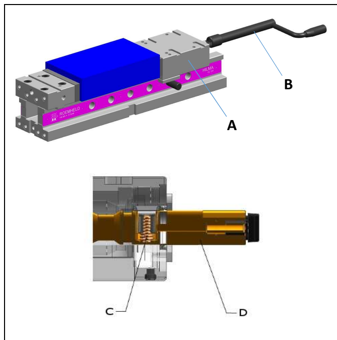
Fig. 5 : Serrage et desserrage
