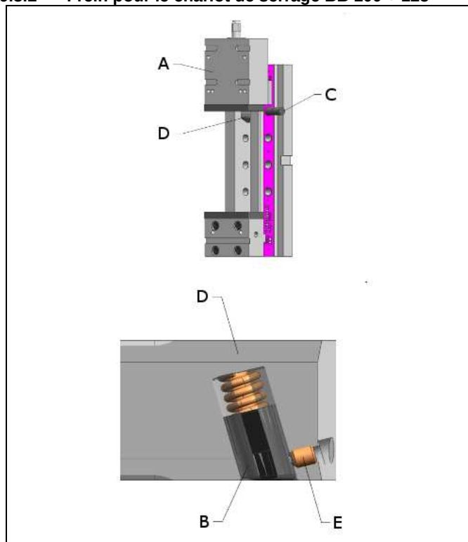
Fig. 6 : Frein pour le chariot de serrage BB 100 + 125
