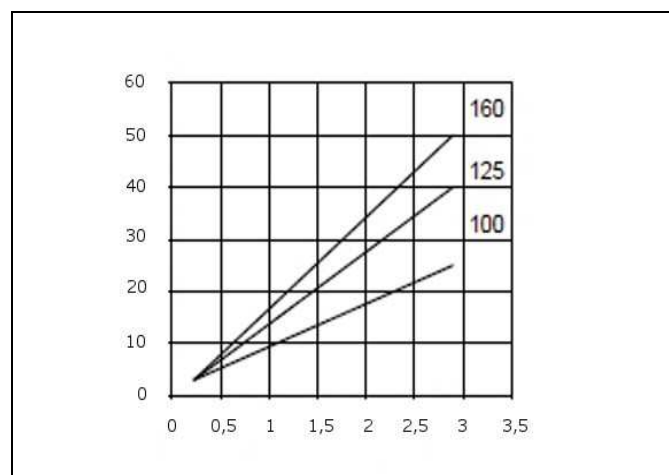
Fig. 11 : Rapports de force de serrage
