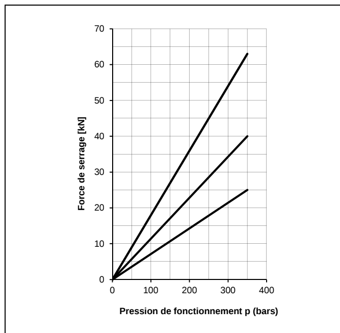
Fig. 9 : Rapports de force de serrage
