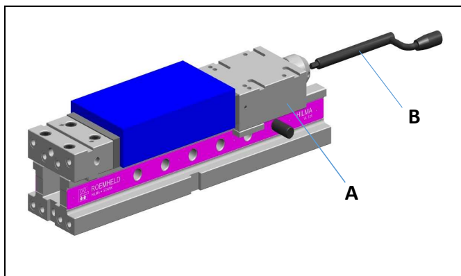
Fig. 6 : Serrage et desserrage
