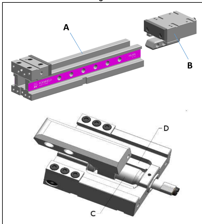
Fig. 8 : Démonter le chariot de serrage
