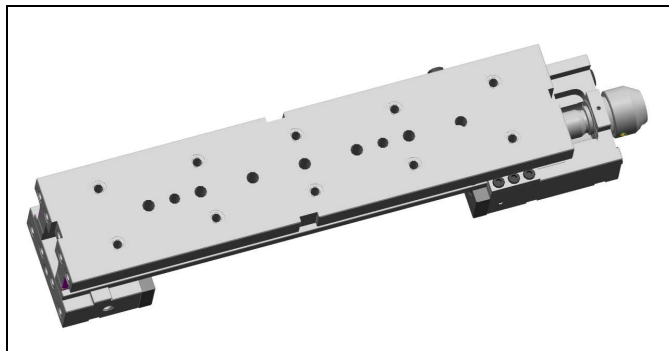
Fig. 3 : Vue de dessous avec alésages de fixation et de positionnement
