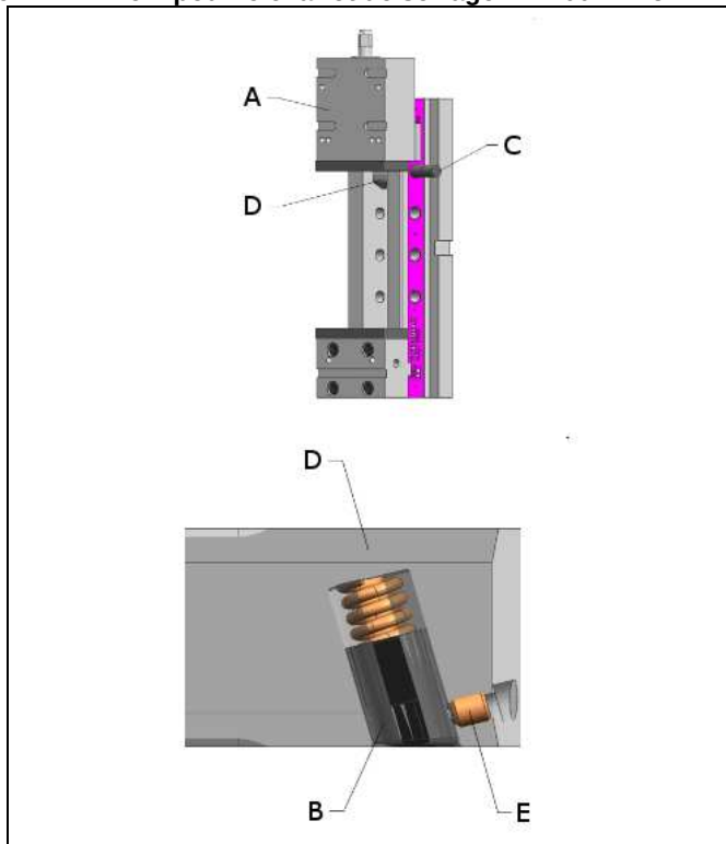
Fig. 7 : Frein pour le chariot de serrage BB 100 + 125
