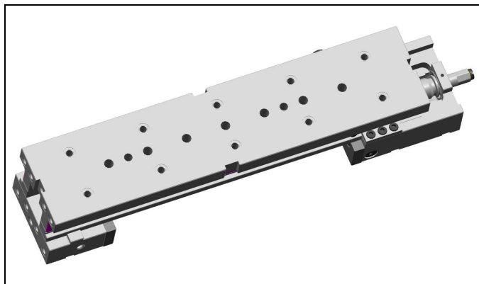
Fig. 3 : Vue de dessous avec alésages de fixation et de positionnement
