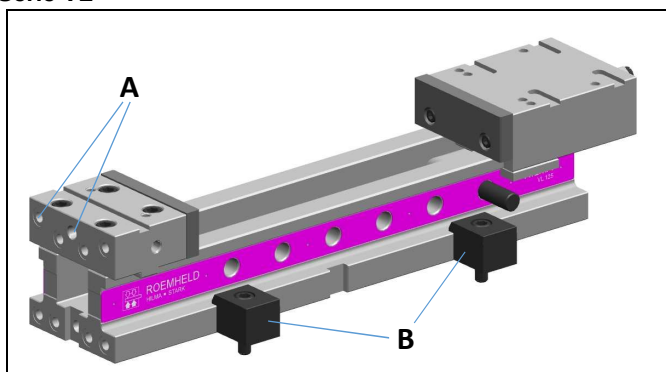
Fig. 2 : Types de montage pour la série VL
