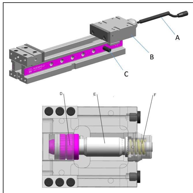
Fig. 1 : Composants pour la série VL
