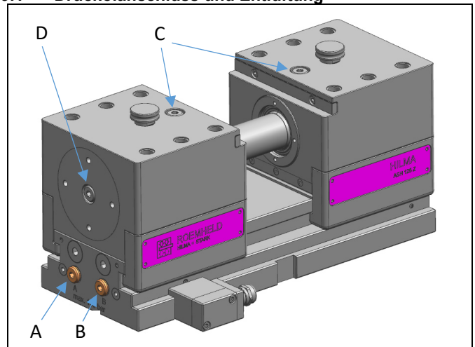
Abb. 11: Druckölanschluss und Entlüftung
