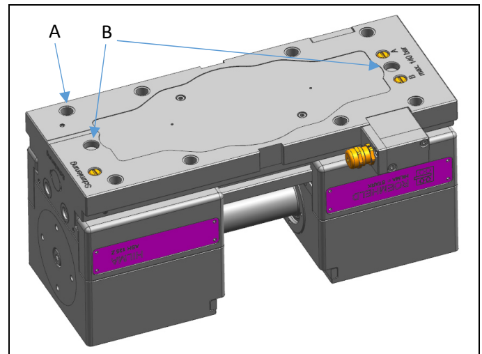
Abb. 2: Montagearten
