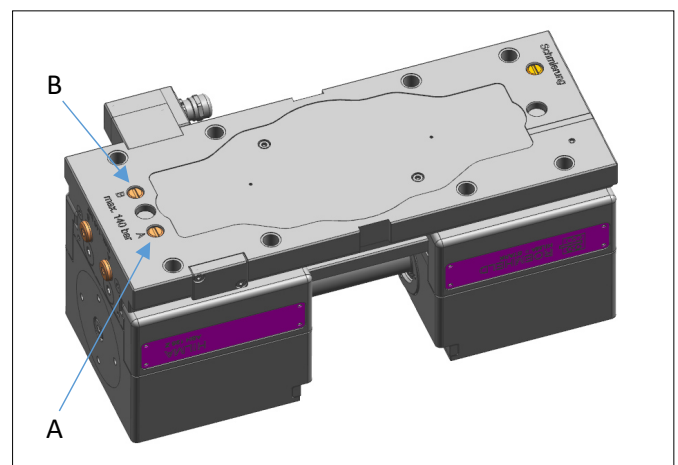
Abb. 12: Druckölanschluss von unten, Drehgeber
